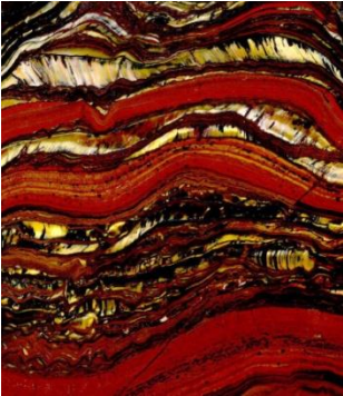
Stromatolites
